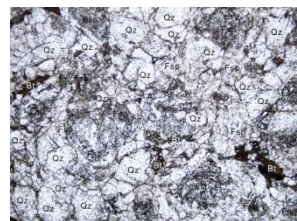
花岗岩显微图 Granite Microscopic Texture
